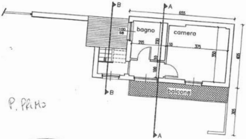
PIANO PRIMO S Scala 1:100
